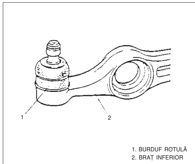
FIG. 3 – 19 INSPECȚIA ARTICULAȚIEI
