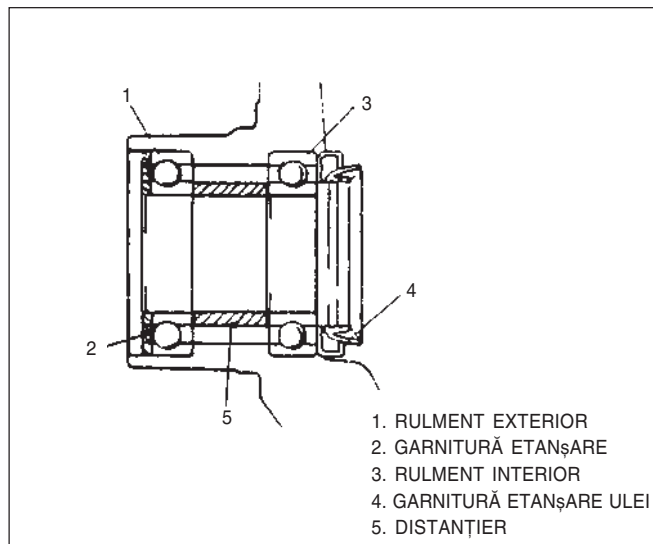
FIG. 3 – 17 BUTUCUL ROȚII
