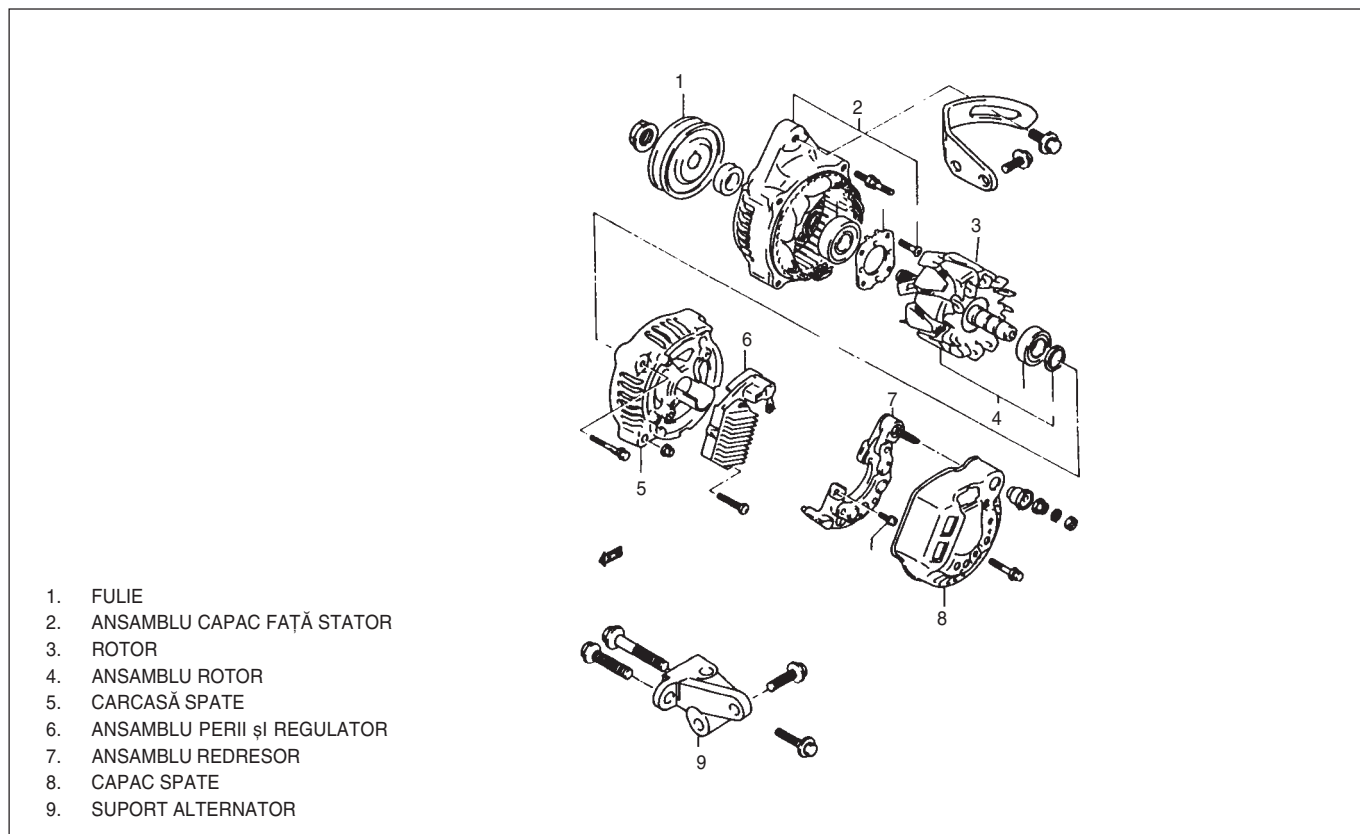
FIG. 6H - 2 ALTERNATOR
