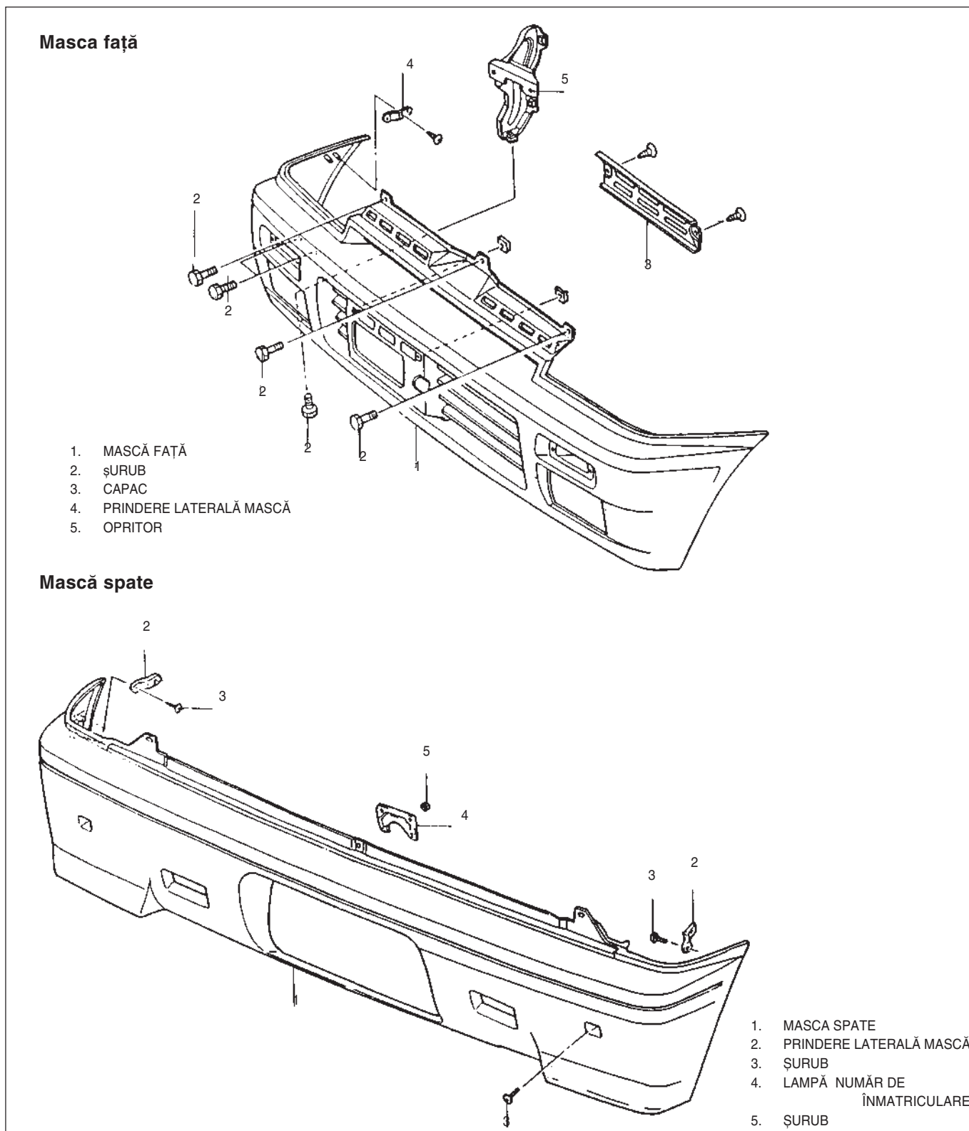
FIG. 12B - 1 MASCĂ FAȚĂ, SPATE
