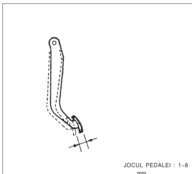
FIG. 5 – 22 INSPECTAREA JOCULUI PEDALEI DE FRÂNĂ
