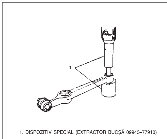
FIG. 3 – 18 EXTRACȚIE BUCȘĂ
