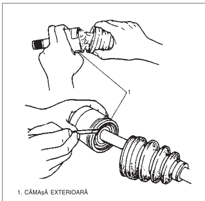
FIG. 3 – 25 DEMONTAREA CĂMAȘII EXTERIOARE
