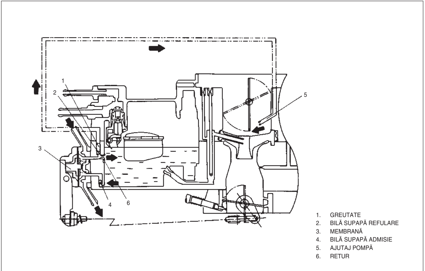
FIG. 6E – 12 POMPA DE ACCELELAȚIE
