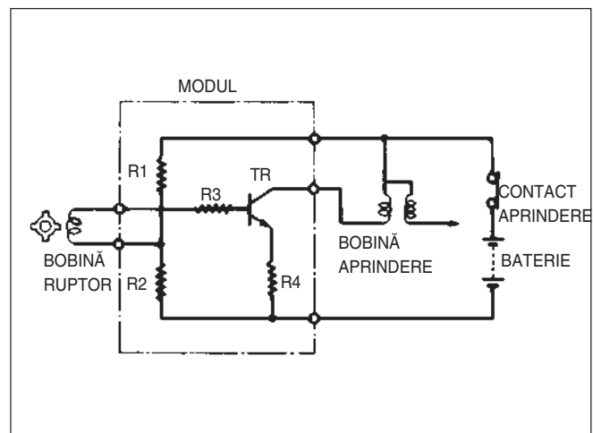
FIG. 6F – 13 CIRCUITUL DE BAZĂ AL SISTEMULUI DE APRINDERE CU COMANDA UNGHIULUI DE ÎNCHIDERE A CAMEI
