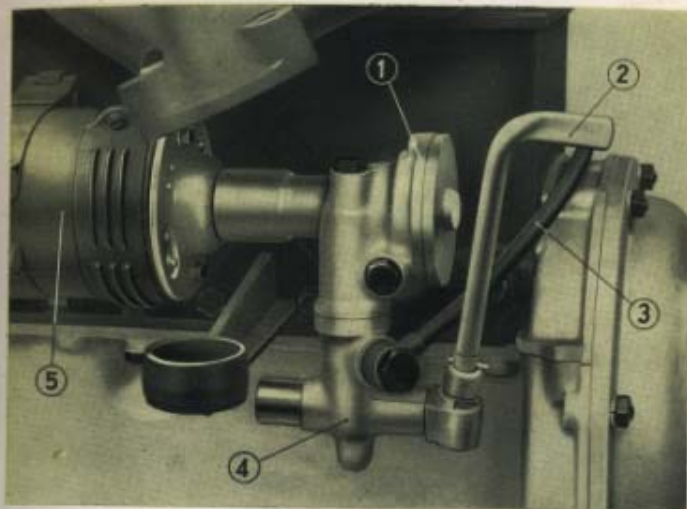
Fig. 23. Pompa acqua e rubinetto scarico acqua del radiatore ed al motore.
