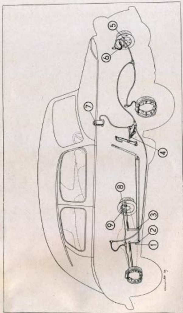
Fig. 39. Schema dell'installazione dei freni.
