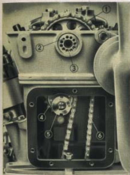
Fig. 12. Messa in fase delle distribuzioni.
