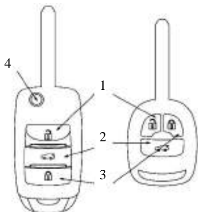
Основной ключ
