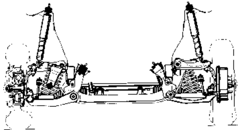
senza barra stabilizzatrice (berlina o coupé)
