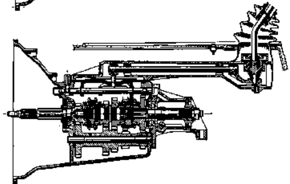
Cambio meccanico con leva corta.
