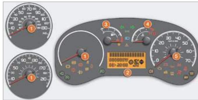
Панель приборов с дисплеем уровня 2
